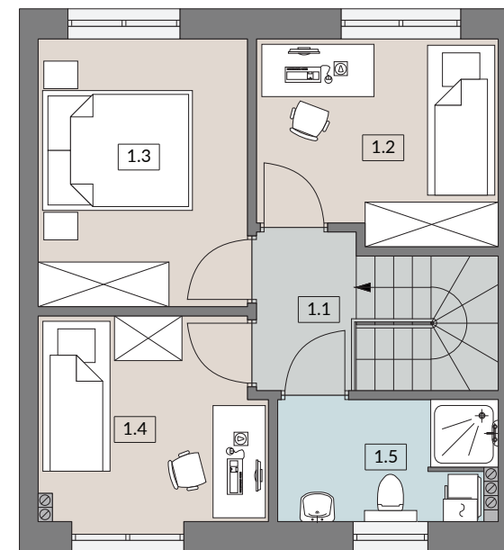
RZUT PIĘTRA
