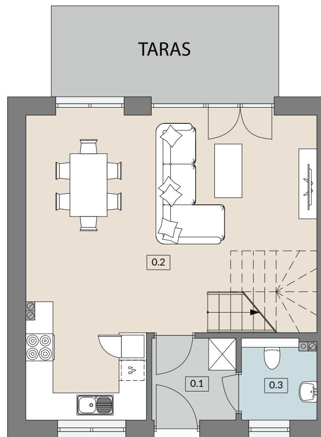
RZUT PARTERU
