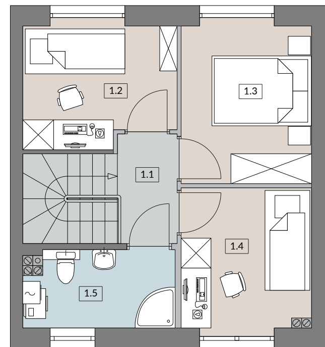
RZUT PIĘTRA
