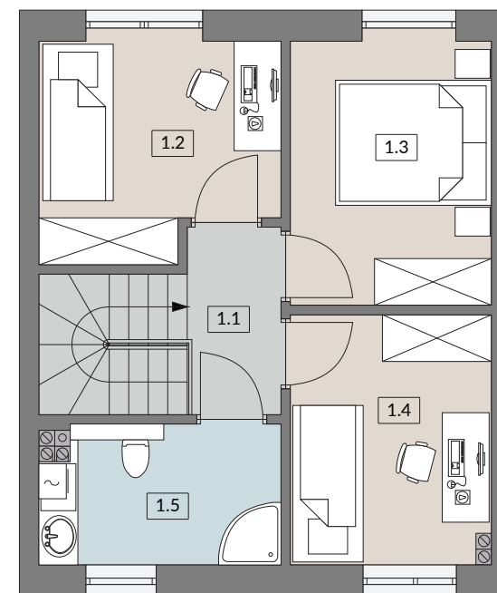
RZUT PIĘTRA
