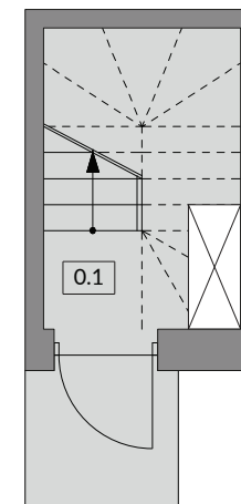
RZUT PARTERU
