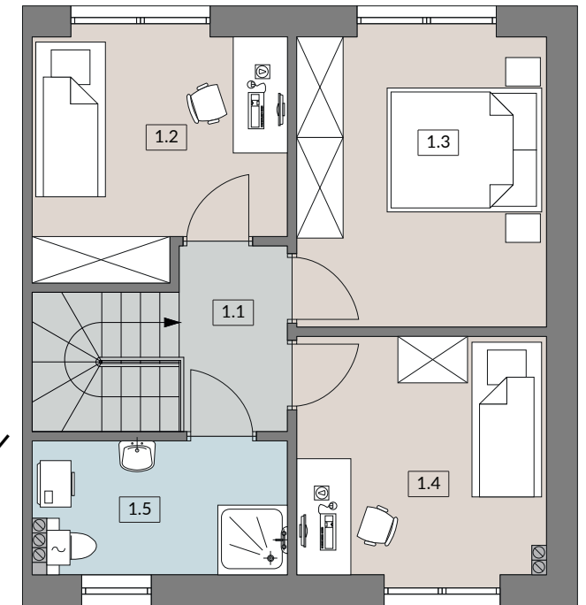
RZUT PIĘTRA
