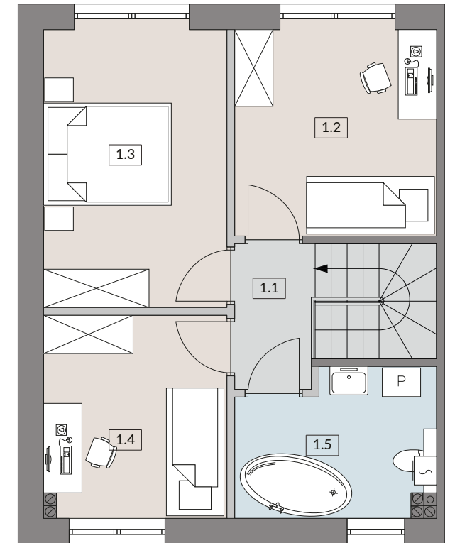
RZUT PIĘTRA
