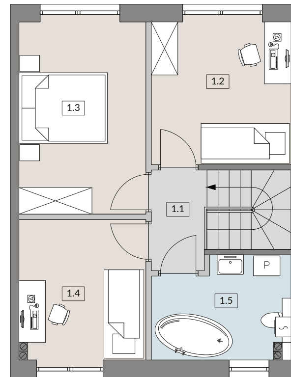
RZUT PIĘTRA
