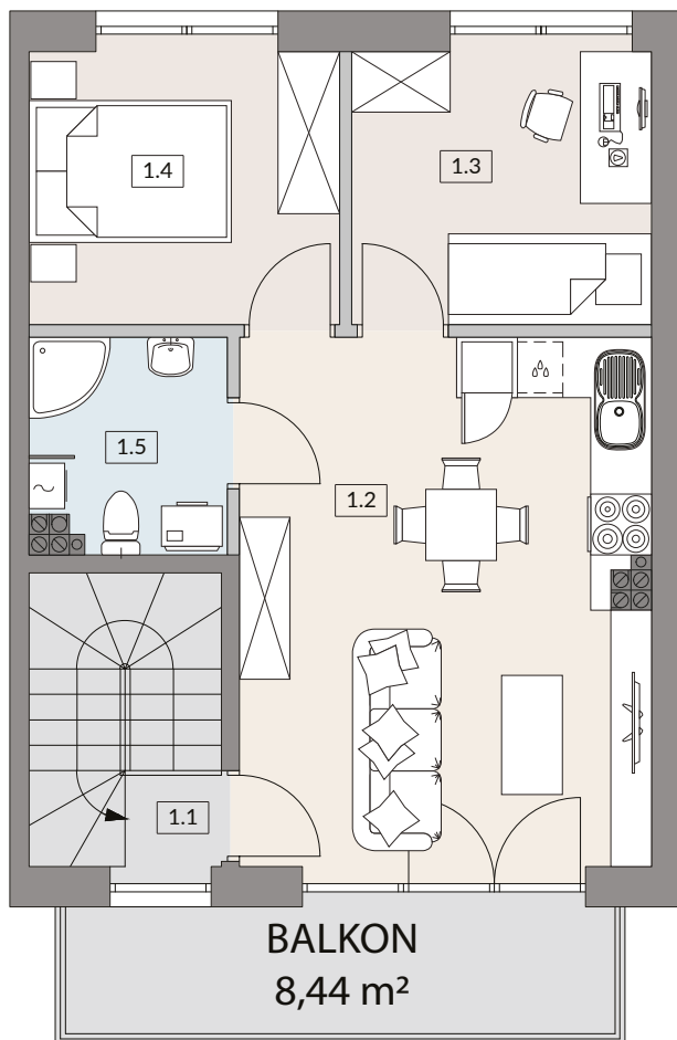
RZUT PIĘTRA
