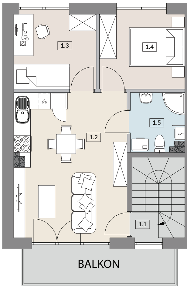
RZUT PIĘTRA
