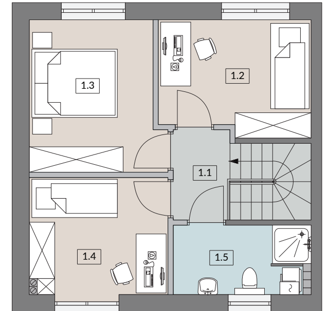
RZUT PIĘTRA
